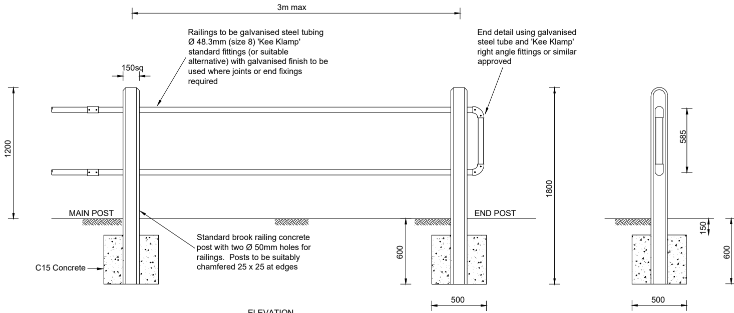
ELEVATION
